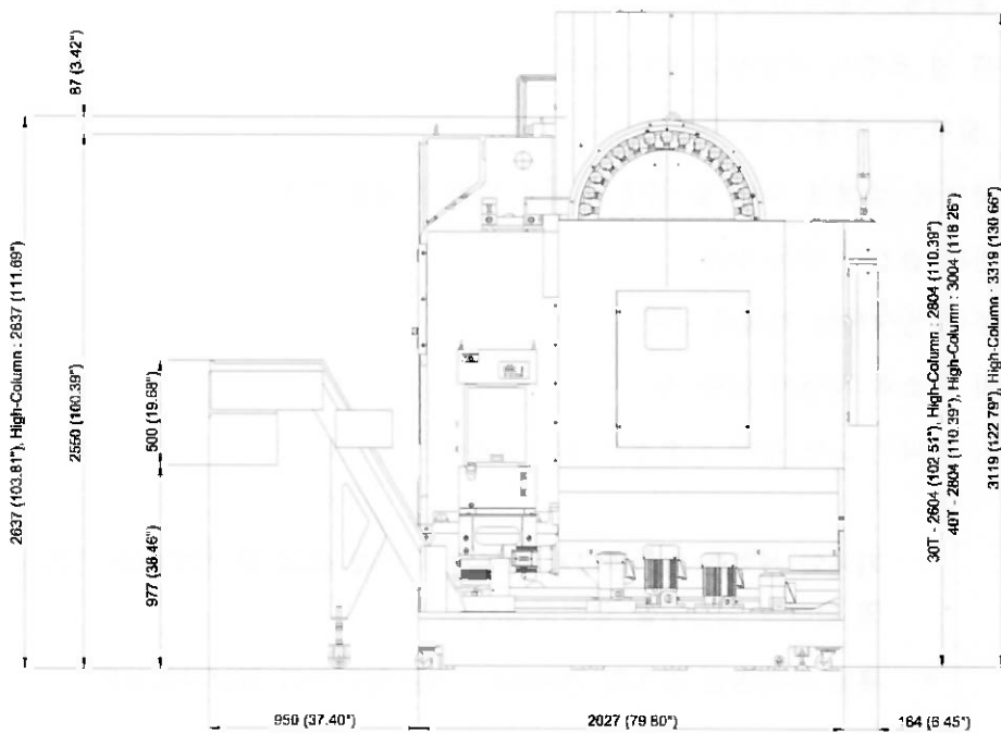
그림 1.4 외형 치수도 (단위: mm (inch))
